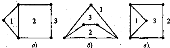
Рис. 25. Грани плоского графа
