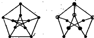
Рис. 27. Граф Петерсена и его подграф, гомеоморфный K_{3,3}
